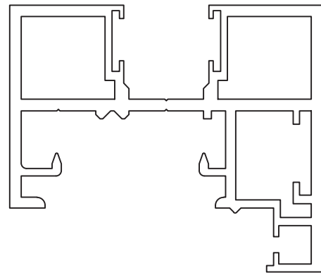
KOZIJN ENKEL GLAS 5-8310
