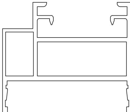
Staander openslaande deur 5-8410
