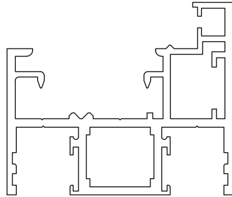
KOZIJN DUBBEL GLAS 5-8320
