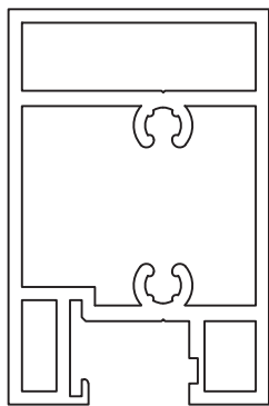
Staander schuifdeur 5-8450
